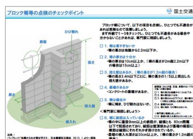
【図 3-11】ブロック塀のチェックポイント
