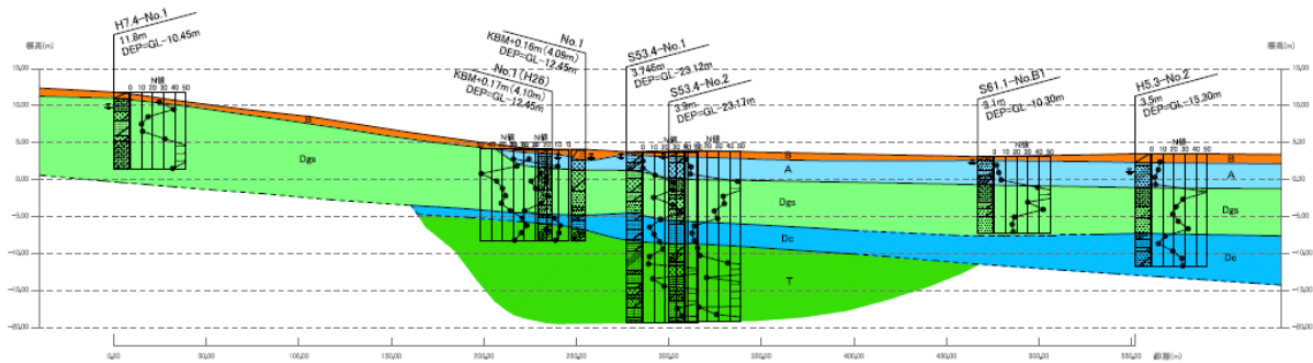
地層推定断面図 (縮尺H=1:2,000, V=1:500)
