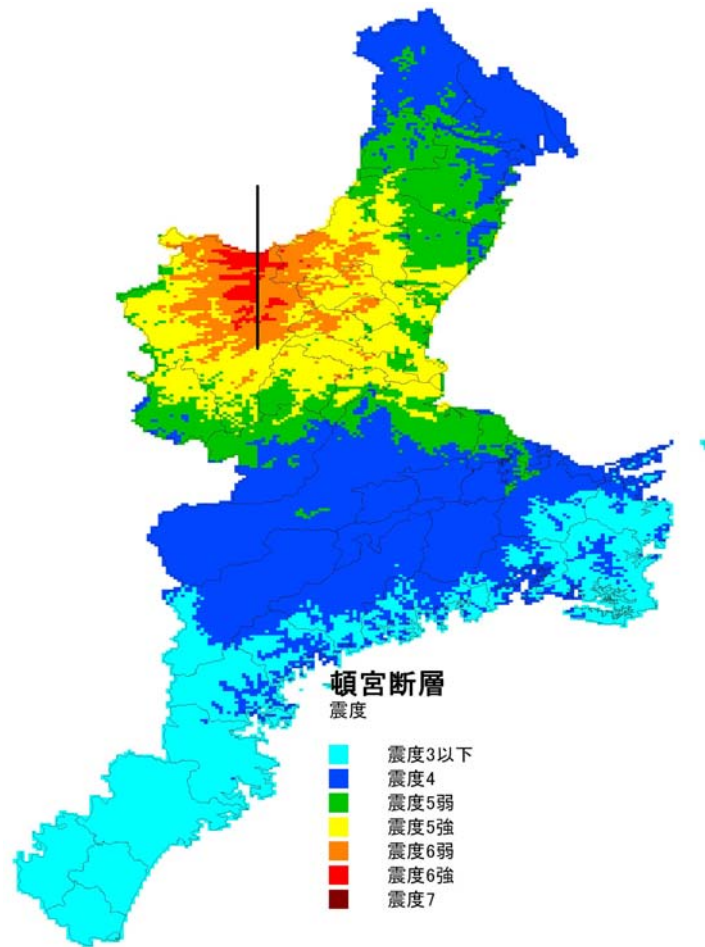
図1 頓宮断層による震度分布
