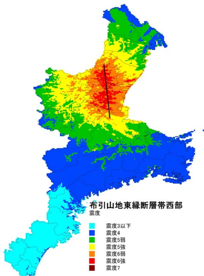
図1 布引山地東縁断層帯西部による震度分布
