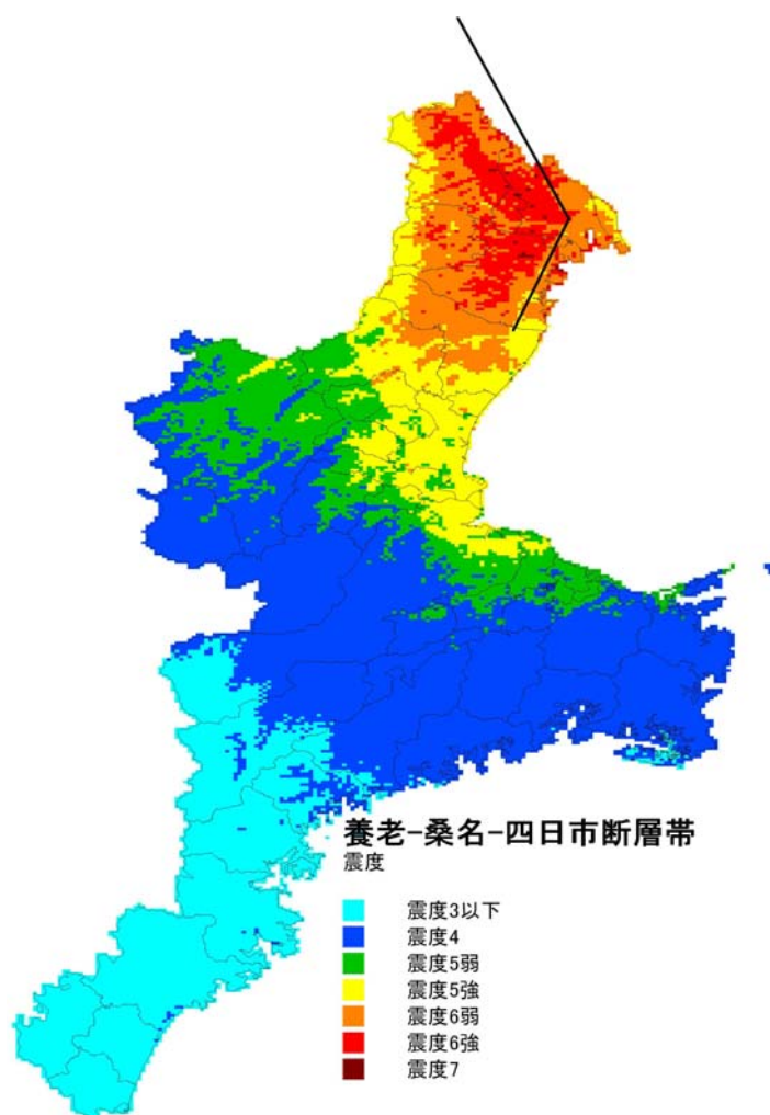
図1 養老-桑名-四日市断層帯による震度分布
